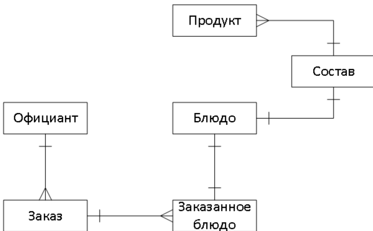
Рис. 3 — Модель данных
